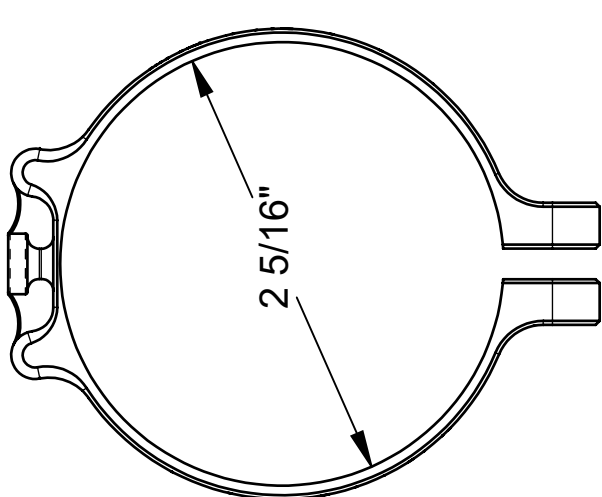
FORK RING (ACTUAL SIZE)
